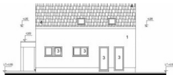
pohled západní
